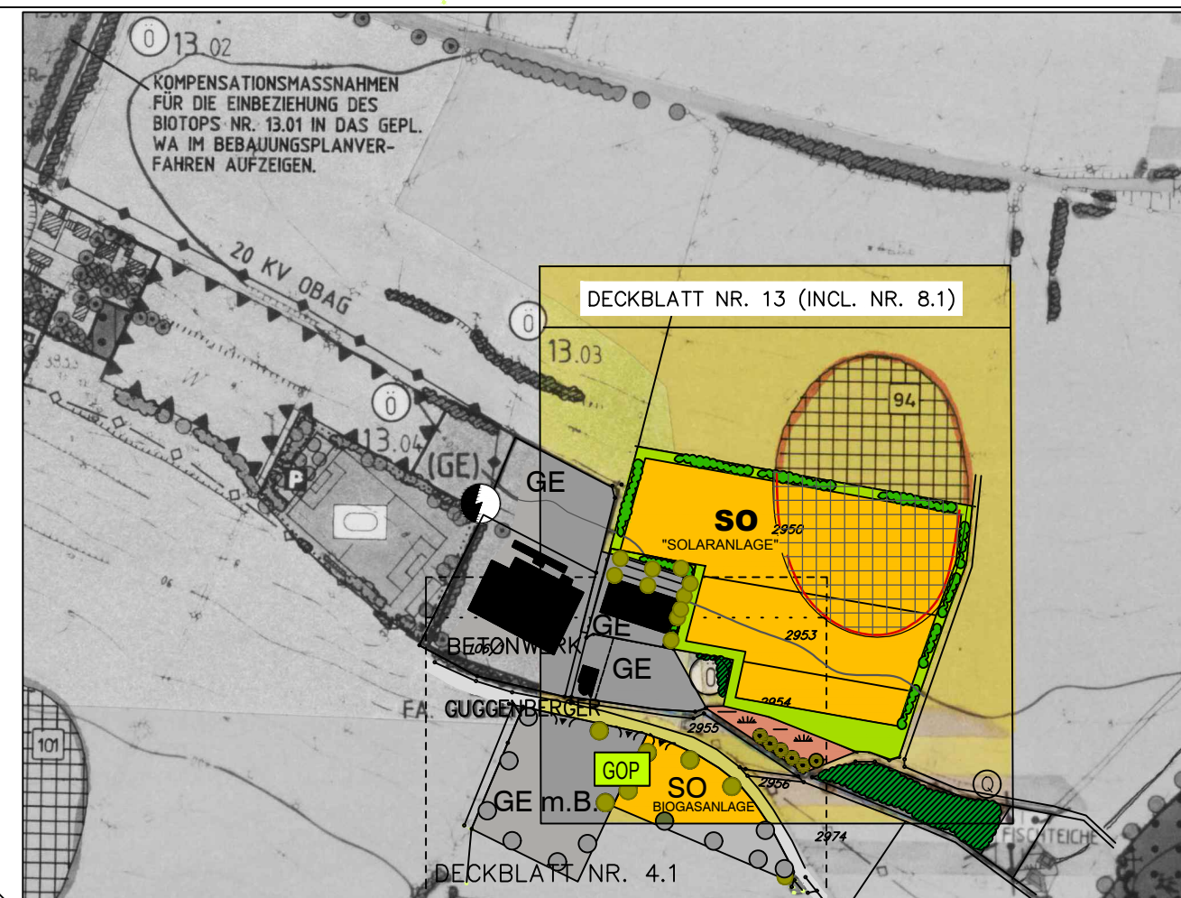
DECKBLATT NR. 13 (INCL. NR. 8.1)
